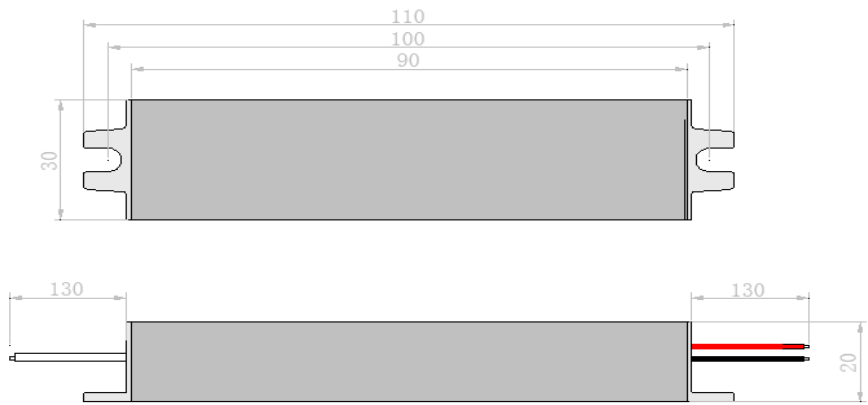
安装尺寸(单位:mm) Configuration dimensions(Unit:mm)
