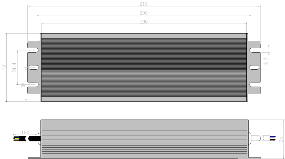
安装尺寸(单位:mm) Configuration dimensions(Unit:mm)
