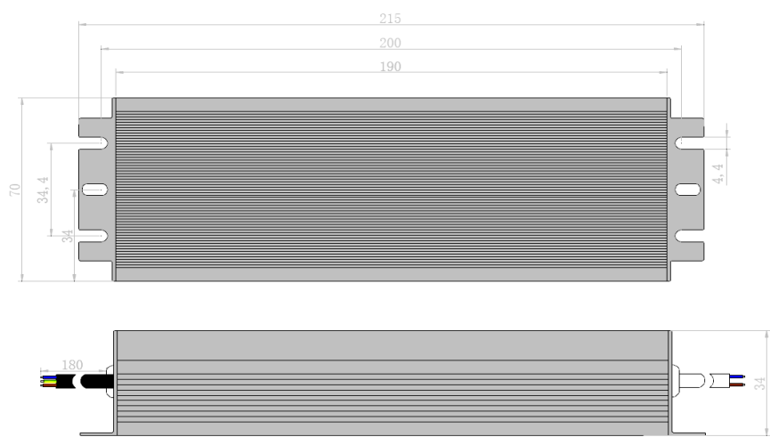
安装尺寸(单位:mm) Configuration dimensions(Unit:mm)
