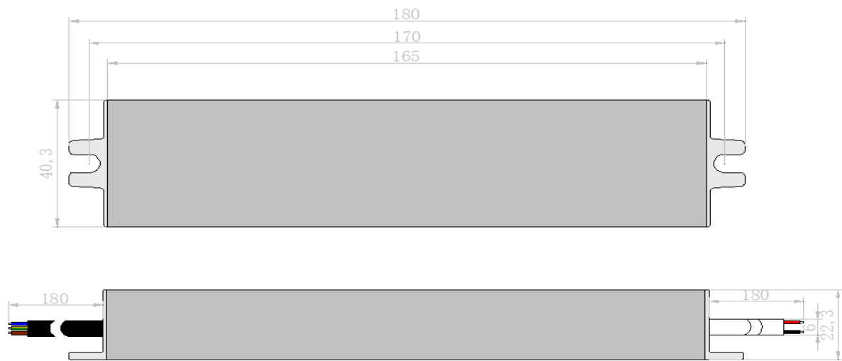
安装尺寸(单位:mm) Configuration dimensions(Unit:mm)
