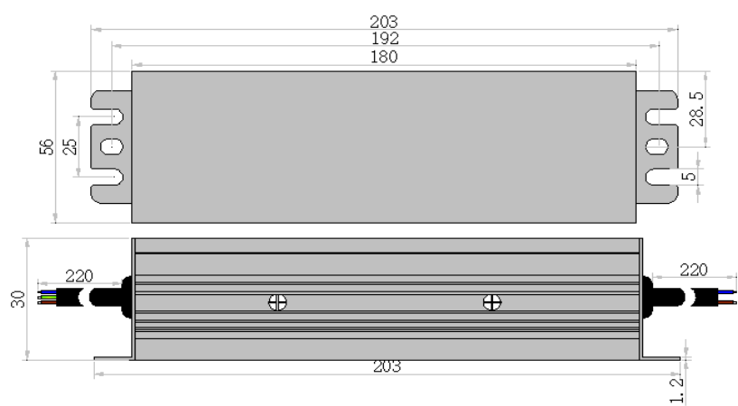
安装尺寸(单位:mm) Configuration dimensions(Unit:mm)
